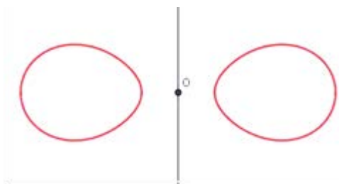
due ovali una esterna all'altra
