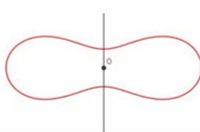
una sola "ovale"
