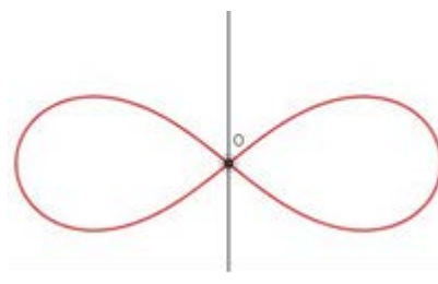
un punto doppio
