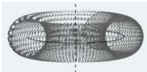
Toro aperto: d > r
